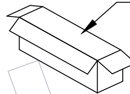
No: 4 内箱内需套防水袋PE-20 真空管装入内箱(3扎/内箱) 内箱规格: CTN-10A(双坑A=B 63*15*17CM)
