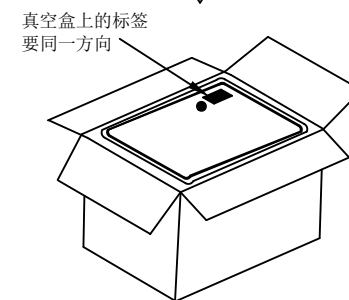
No. 4: 纸箱内需套防水袋PE-19, 加两包干燥剂, 再装真空盒装入纸箱 (11盒/箱, 共385PCS/箱) 纸箱规格: CTN=74 (双坑K=K, 30.5*30*33.5cm)
