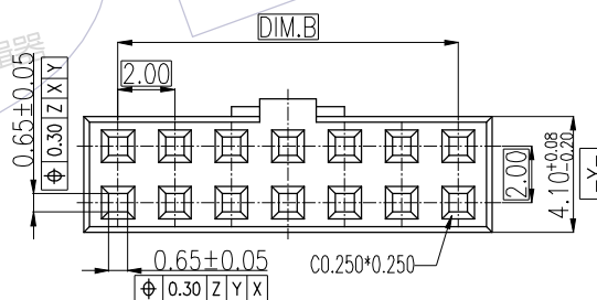
DETAIL:B-B SCALE:1/1
