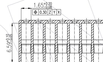
DETAIL:B-B SCALE:1/1
